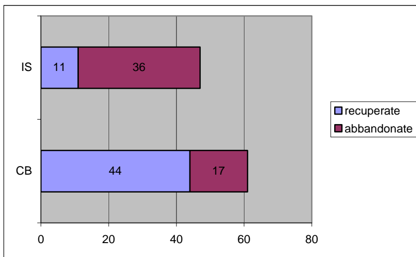
FIG. 3.6 – Attività estrattive abbandonate e recuperate
