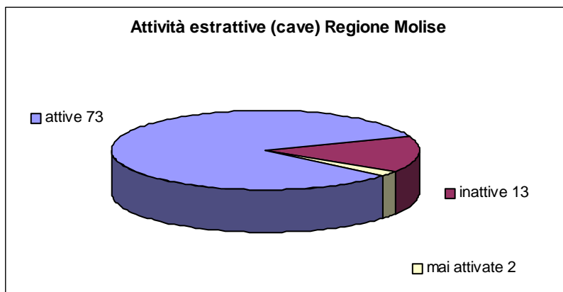
FIG. 3.2 – Numero cave e attività estrattive in esercizio, inattive o mai attivate
