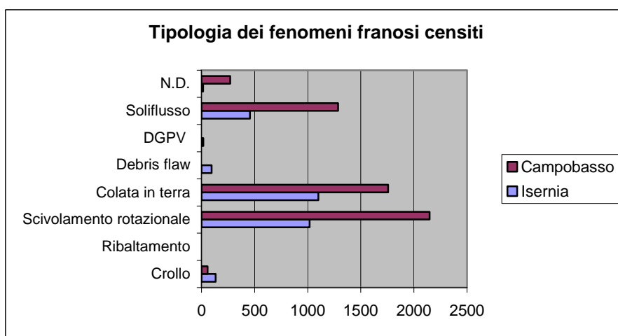
FIG. 3.9 - Tipologia dei fenomeni franosi censiti (per provincia)
