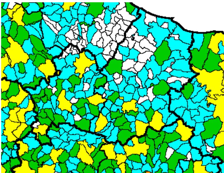
FIG 3. 14 - Danno totale annuo atteso del patrimonio abitativo per comune (metri quadri equivalenti)
