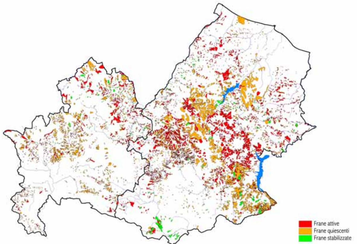
FIG. 3.7 – Territorio interessato da frane attive, quiescenti e stabilizzate con riferimento al sistema idrografico
